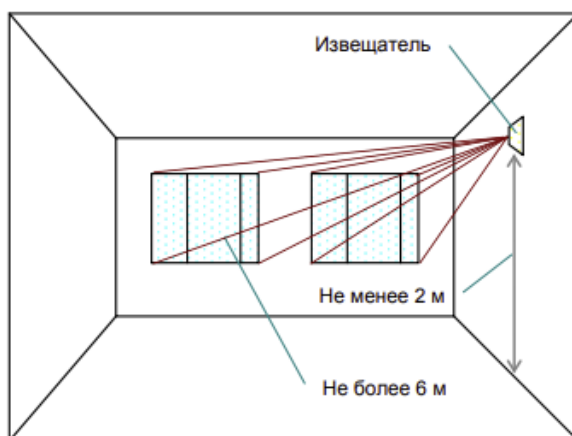
Установка извещателя на боковой стене
