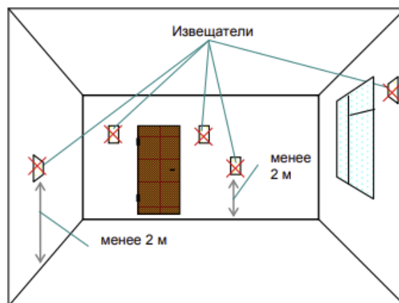
НЕрекомендуемые места установки извещателя
