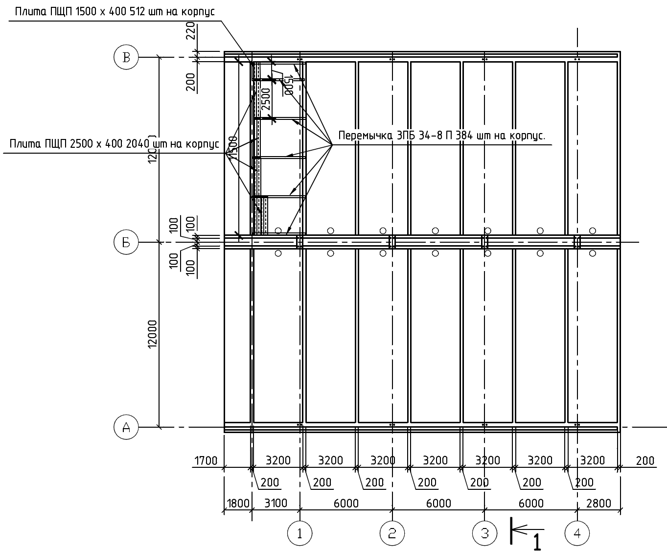
Схема укладки перемычек и щелевых плит СВК Рождественка корпуса 3 и 4
